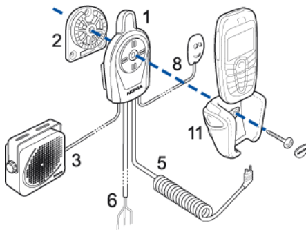
Zestaw samochodowy z pasywnym uchwytem do telefonu
