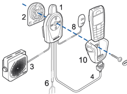
Zestaw samochodowy z aktywnym uchwytem do telefonu
