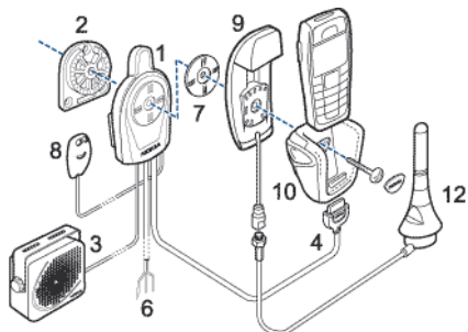
Zestaw samochodowy z oddzielnym adapterem antenowym i zewnętrzną anteną
