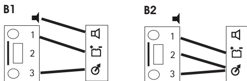
Načini vgradnje s stereo zvokom
