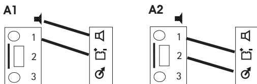
Načini vgradnje z mono zvokom
