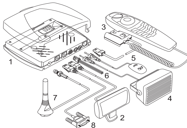
Συνδέσεις εξοπλισμού και καλωδιακές συνδέσεις στο τηλέφωνο αυτοκινήτου
