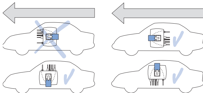
Εγκατάσταση της μονάδας ραδιοφώνου στο αυτοκίνητο
